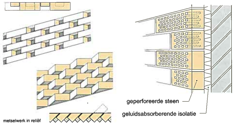
Figuur 24. Geluidsabsorberende oplossingen in metselwerk
