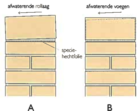
Figuur 17. Afdekking metselwerk met gemetselde rollaag
