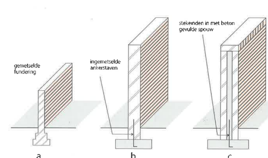
Figuur 2 Vrijstaande muren zonder penanten.
