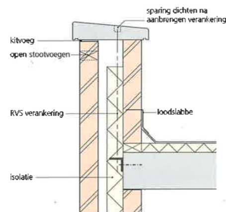
Figuur 17 Detailering dakrand met boekprofiel en ankerstaaf.
