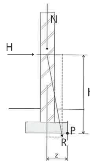
Figuur 1 Stabiliteit van de fundering tegen kantelen is gewaarborgd als N \cdot z / H \cdot h \geq 2
