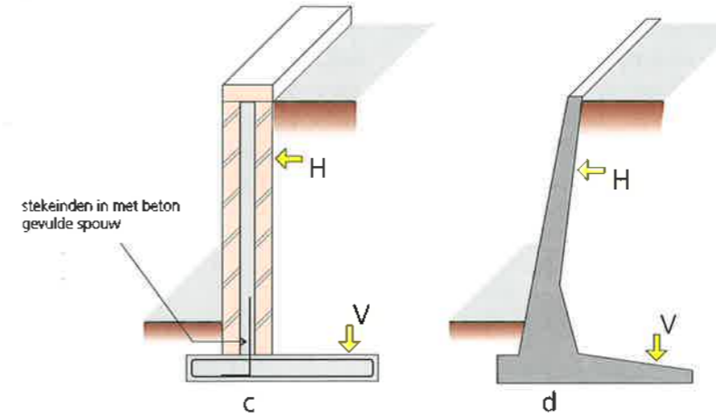
Figuur 25 Diverse typen keermuren.
