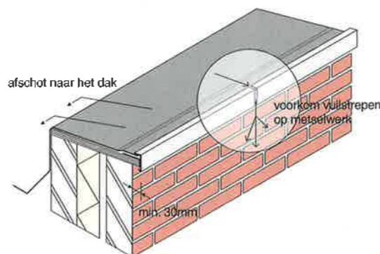
Figuur 29 Borstwing bovendaks moet goed afwateren naar het dak om vuilsporen op de gevel te plaatsen van de naden in de daktrim te voorkomen.
