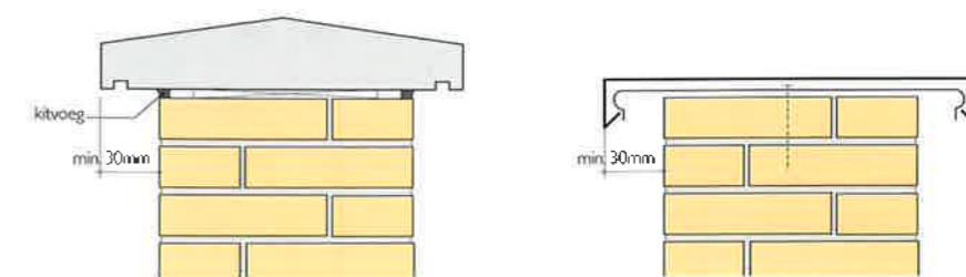
Figuur 37 Prefab afdekkingen metselwerk.
