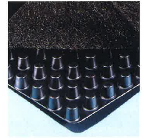
Figuur 26 Drainerende folie, geschikt voor verticale verwerking in funderingen, kelder- en keermuren (Nopbdrain®, Kerkrade).
